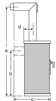
Maß a und c: mit Original-Winkelrohr dimension a and c: with original angle pipe Côtés a et c : avec conduit coude d'origine Wymiary a i c : z oryginalną rurą pod kątem 90°
